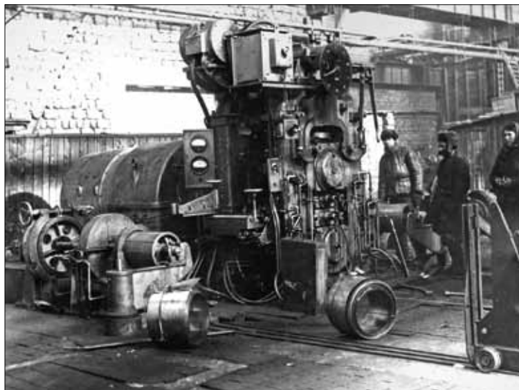
Отделение цеха № 1 Новосибирского металлургического завода. 1942 г.
